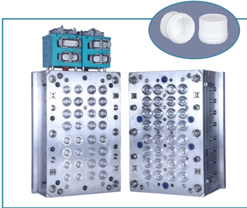
32CV-25MM-ROPP CAP
